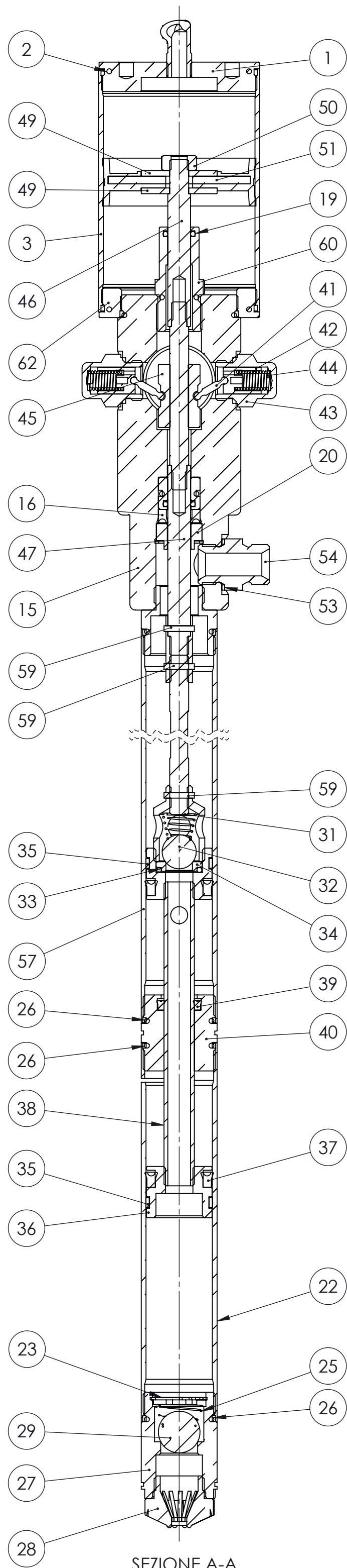
SEZIONE A-A
