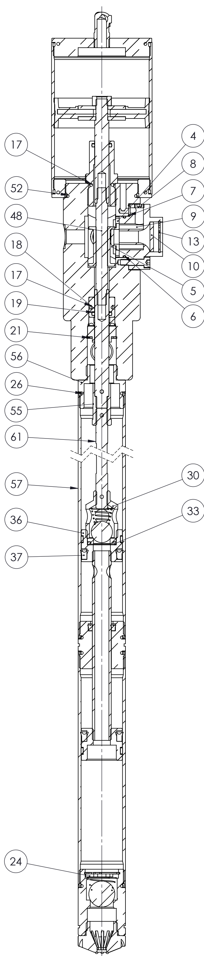
SEZIONE B-B
