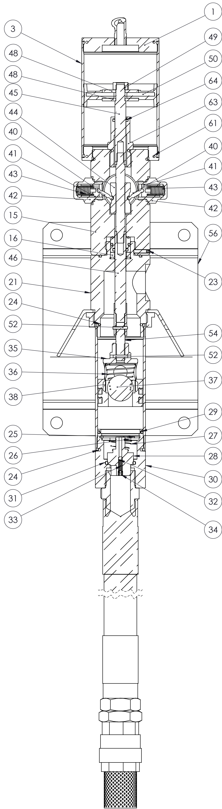
SEZIONE A-A
