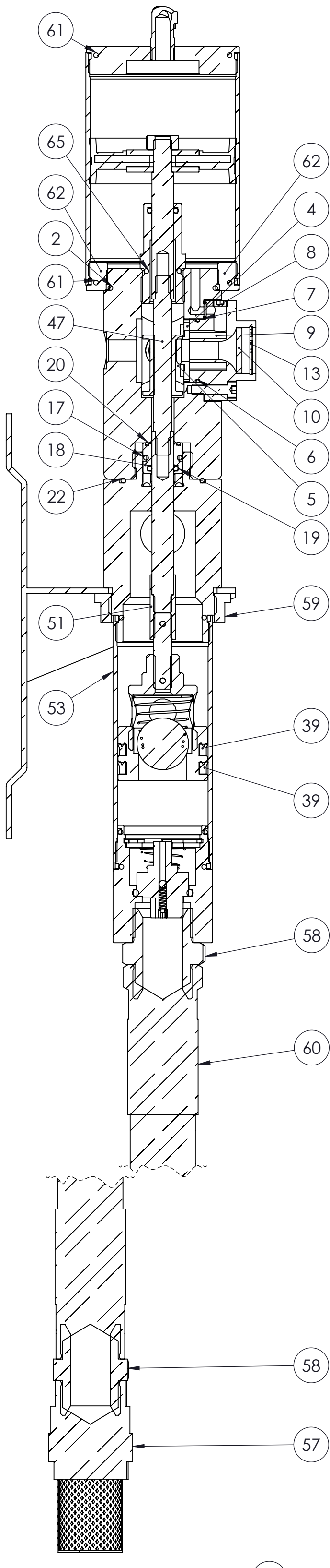
SEZIONE B-B
