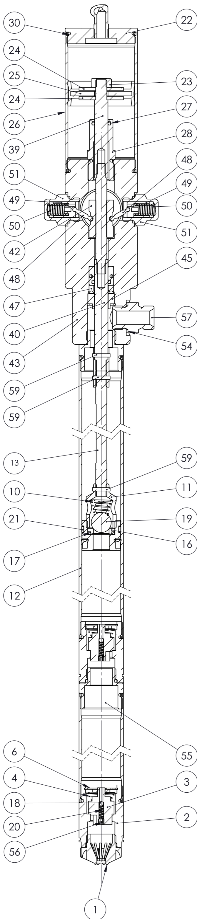
SEZIONE A-A
