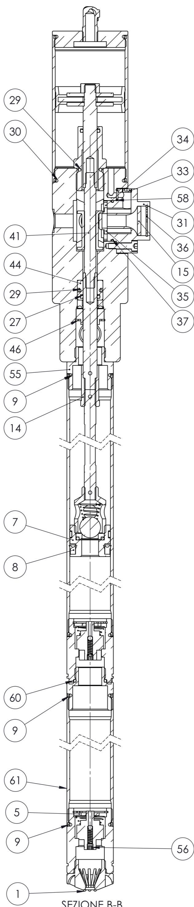
SEZIONE B-B
