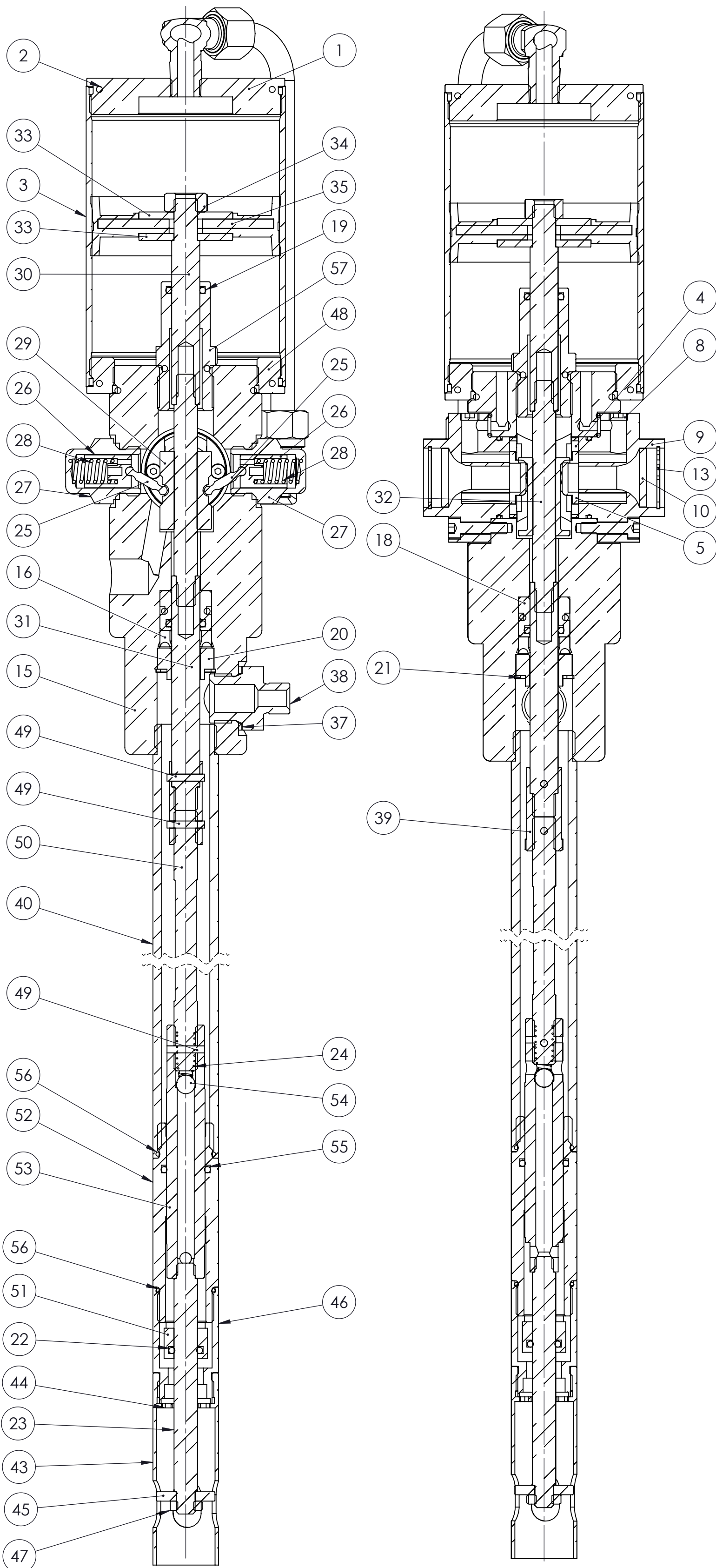
SEZIONE B-B
