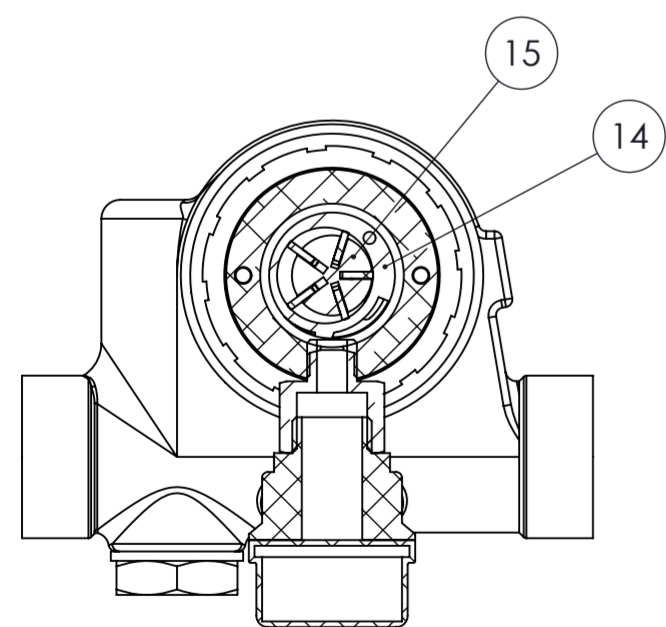
SEZIONE C-C
