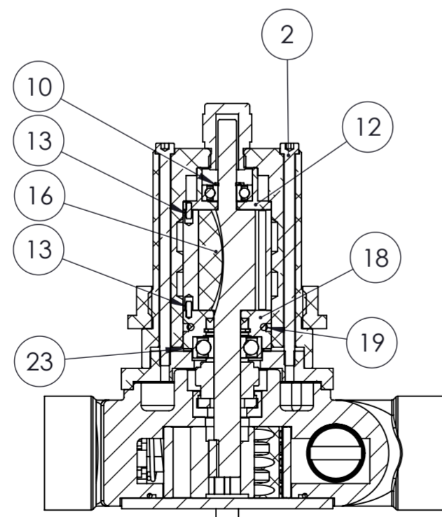
SEZIONE D-D
